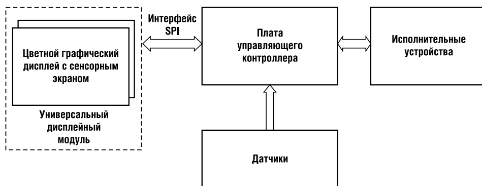
Рис. 1. Структура микроконтроллерной системы с разделением функций отображения и управления
