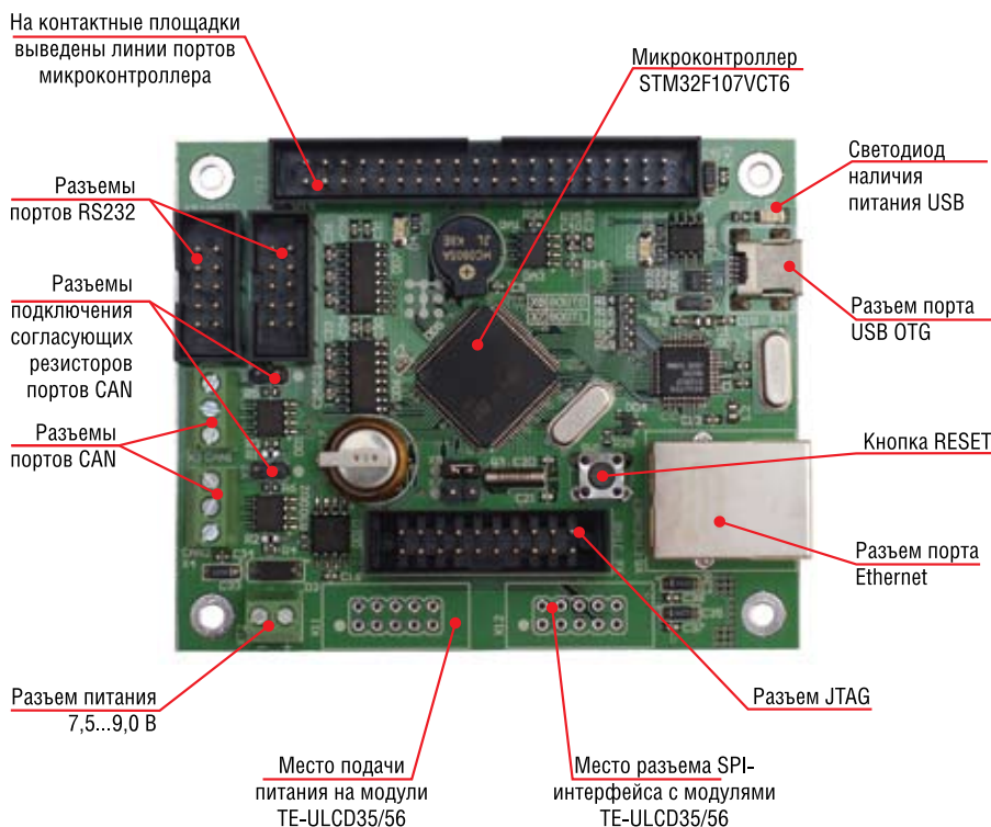
Рис. 3. Микроконтроллерный модуль TE-STM32F107
