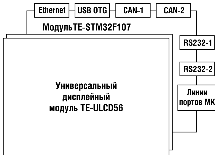
Рис. 5. Интерфейсы системы на основе TE-ULCD35 и TE-STM32F107
